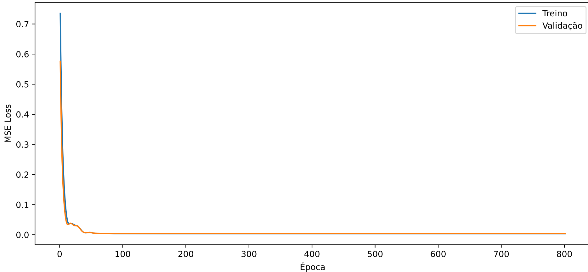
Curva de aprendizagem do neurónio linear em PyTorch
